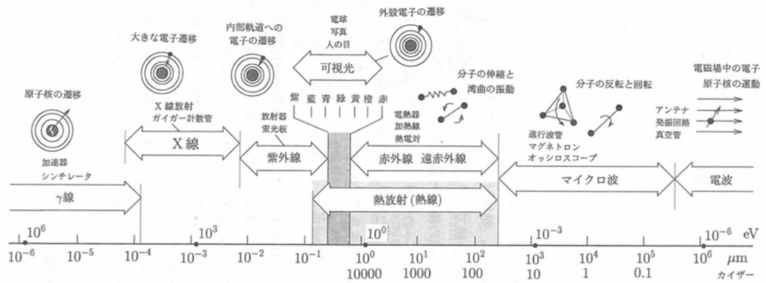
図 10.1 電磁波 (光) の種類
