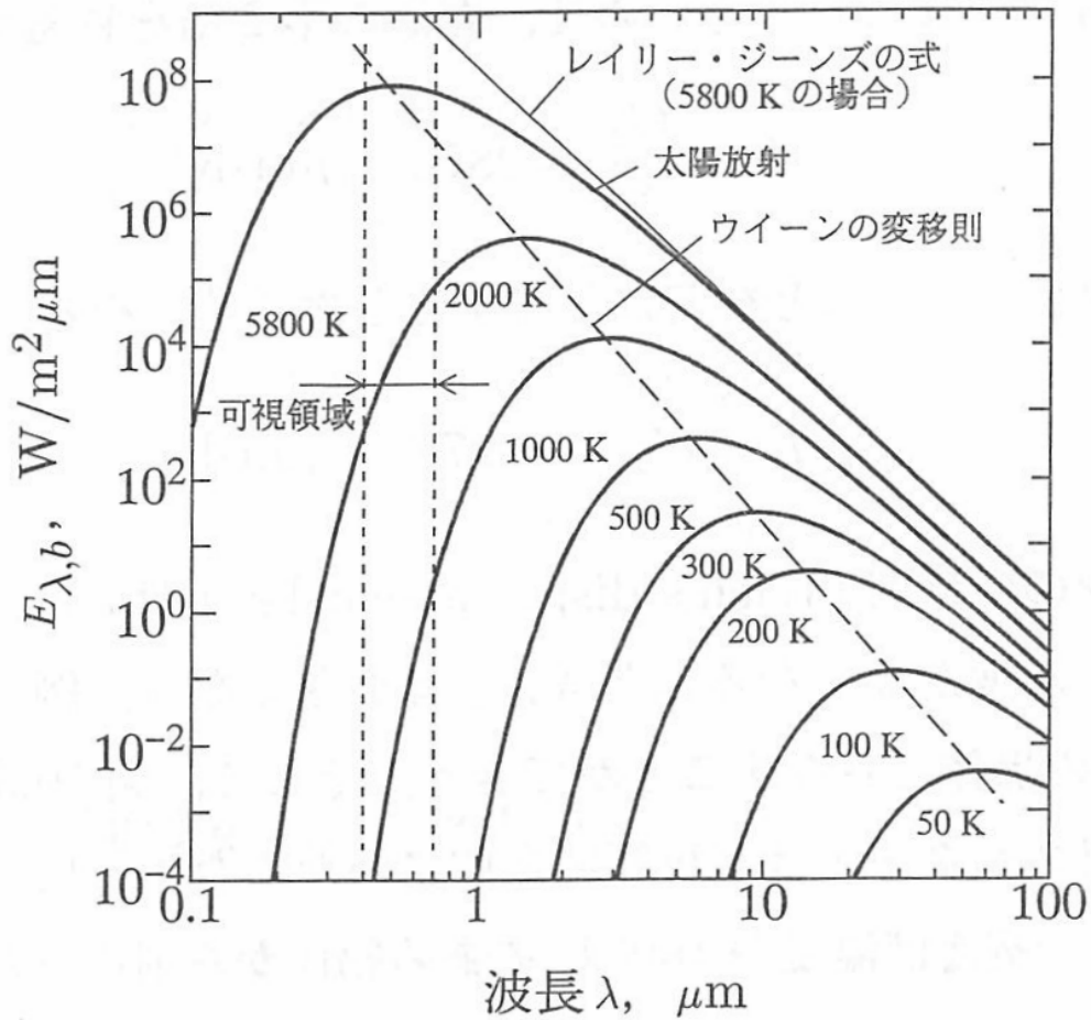
図 10.3 黒体放射 (プランクの式)
